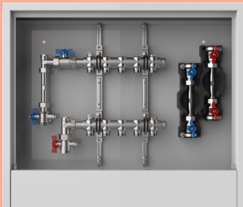
6.1.3 Anschlussstation H 52 im Aufputzschrank A Einbauhöhe von OK FFB 610 mm Bautiefe 125 mm
