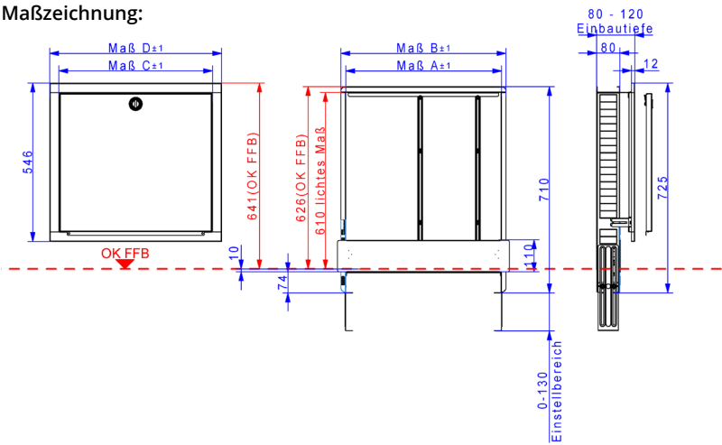
Maßzeichnung:
