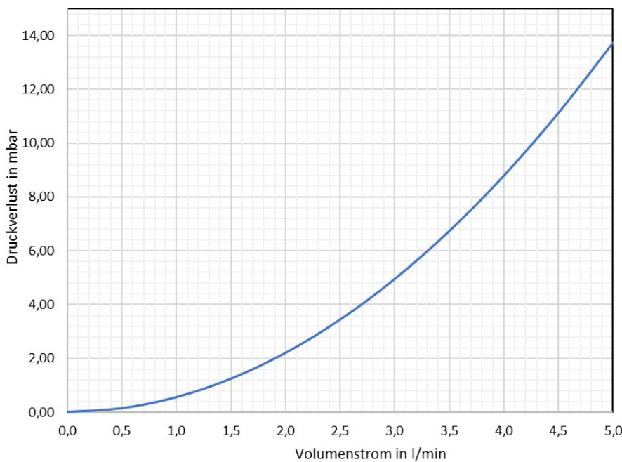
Druckverlustdiagramm Thermostatventileinsatz VA-M30x1,5
