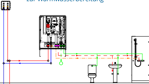
Friwara W-HT zur Warmwasserbereitung + Hochtemperaturabgang für statische Heizflächen (z.B. Heizkörper)
