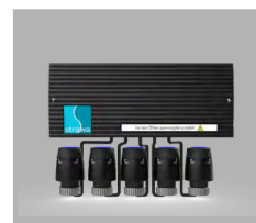
strawalogix RT-STA 230 V und strawatherm 230 V + Vorverdrahtung
