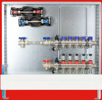
6.1.2 Anschlussstation H 63 im Unterputzschrank 69 Einbauhöhe von OK FFB 640 mm Einbautiefe 110-150 mm
