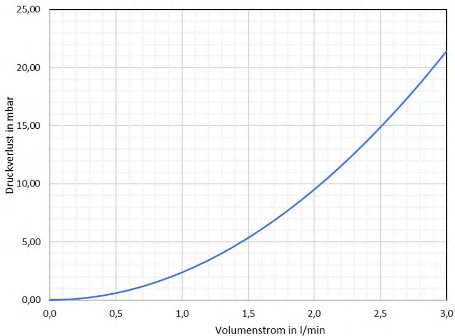
Druckverlustdiagramm Regolux Durchflussanzeiger 0-3 l/min
