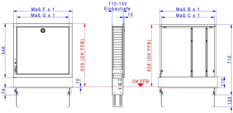
Maßzeichnung:
